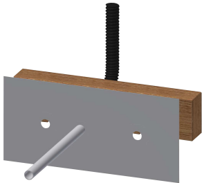
Travesaño de montaje para grifos murales F5
