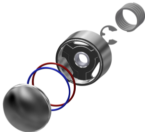
Druckkappe
