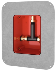
R5 Puszka systemowa do podtynkowych baterii z mieszaczem
